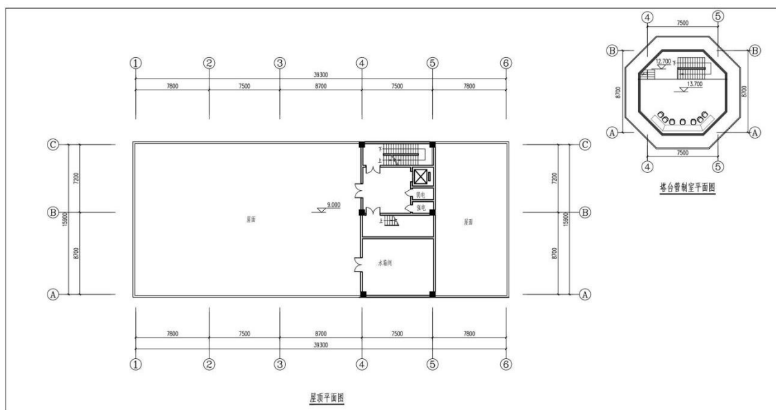
图2-11 综合业务楼屋顶平面及塔台平面图
