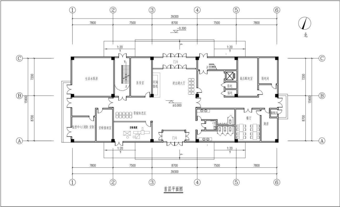
图2-9 综合业务楼一层平面图
