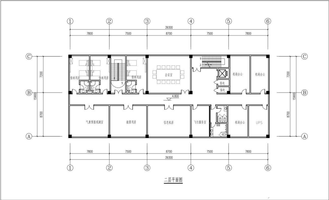
图2-10 综合业务楼二层平面图
