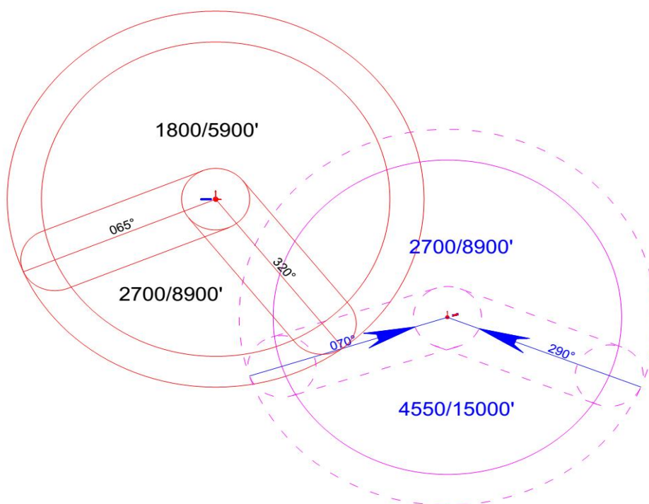
图 2-3 木垒通用机场 MSA 与奇台机场 MSA 位置关系
