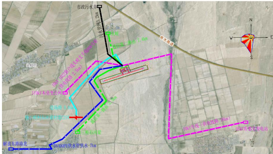
木垒通用机场总体方案布置图
