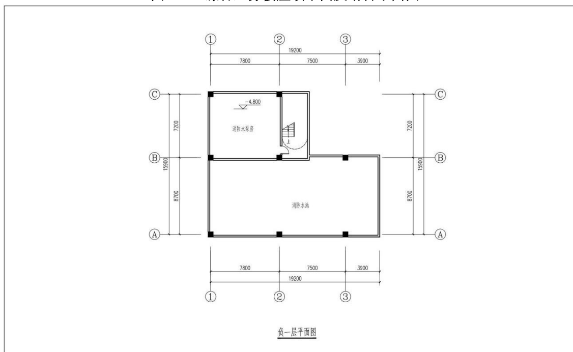
图2-12 综合业务楼负一层平面图
