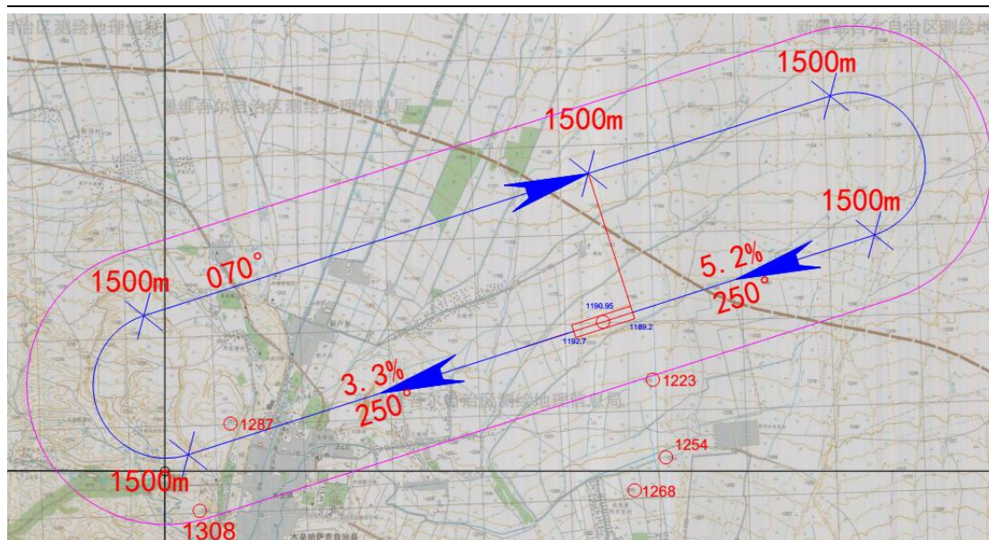
图 2-7 RWY 25 起落航线
