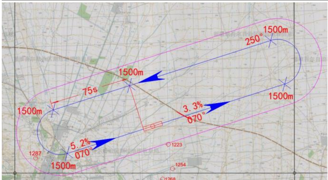
图2-6 RWY07 起落航线
