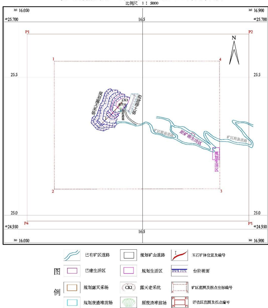
皮山县新藏公路379公里柯里木玉石矿矿山布局平面图
